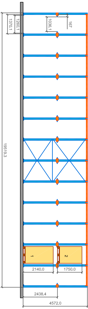
Escala 1: 100 Alzado
